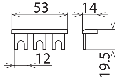
Maßbild MVS 1 3
