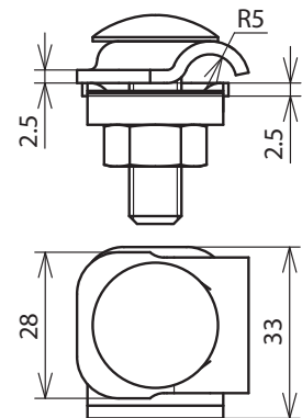
Maßbild MMVK 6.8 FRM10X35 V2A
