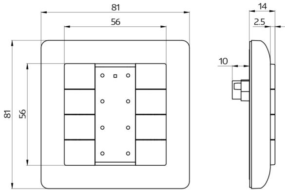
Bemaßung 93178
