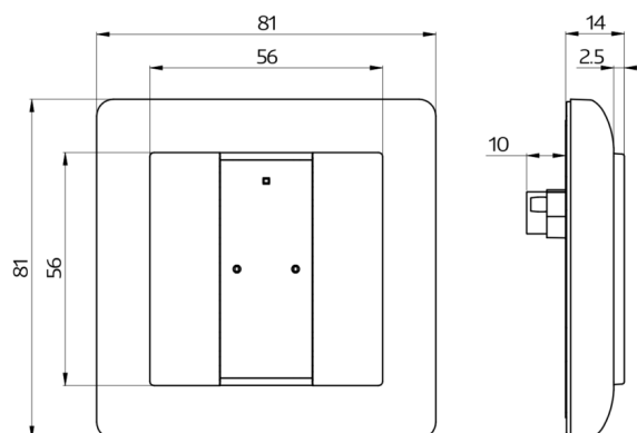
Bemaßung 93172
