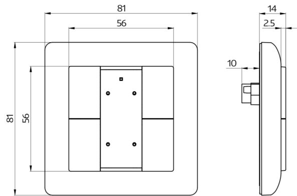
Bemaßung 93174
