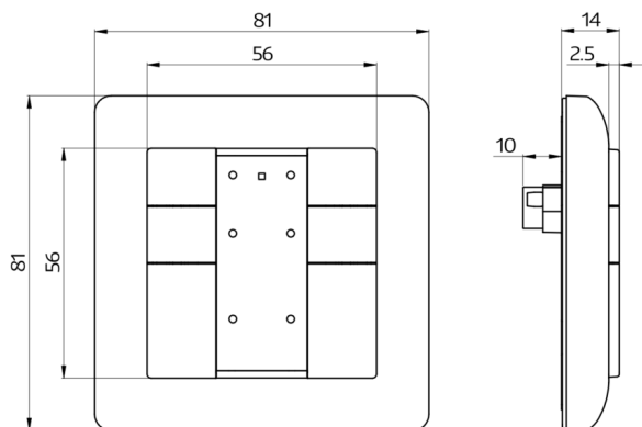
Bemaßung 93176
