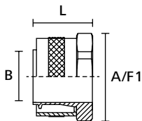
HeliaGuard Verschraubung, Einführungsbuchse
