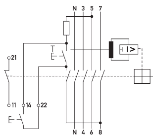
Anschlussschema
