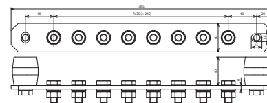
Maßbild PAS I 8AP M10 V2A
