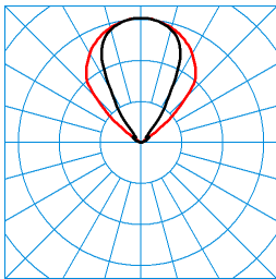
Bicult Act T G2 SMC TGCS 55 ETDI QI 01EU (ACTIWW) TX369882 ■ C0 - C180 ■ C90 - C270 DIN 5040: E04 UTE: 0,00 J + 1,00 T CEN Flux Code: 0 0 0 0 100 82 96 100 100
