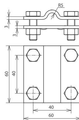
Maßbild KS 8.10 FL30 STTZN
