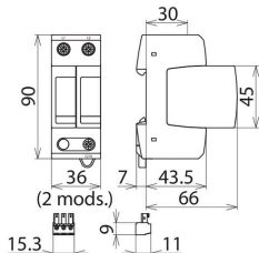
Maßbild DG MU CGD 480 3W+G
