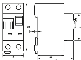
Maßzeichnung Gruppenansicht
