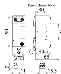
Maßbild DSE M 1 220 FM
