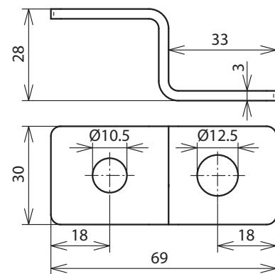
Maßbild ES ZF 2XB18 V2A
