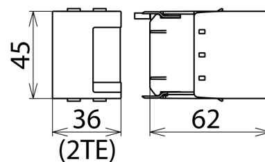
Maßbild DGPH MOD 255
