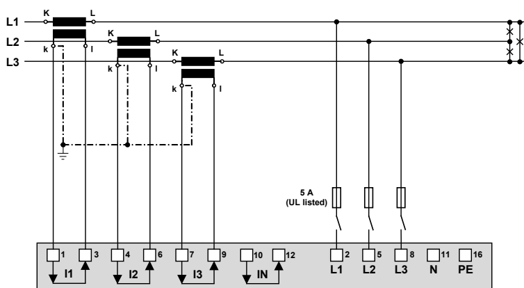
Mit Stromwandlern
