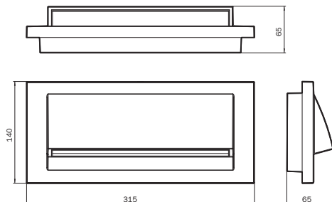
Maße ZAW Dimensions ZAW
