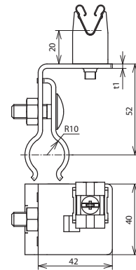
Maßbild DLH DG 8 RSF20.25 AL
