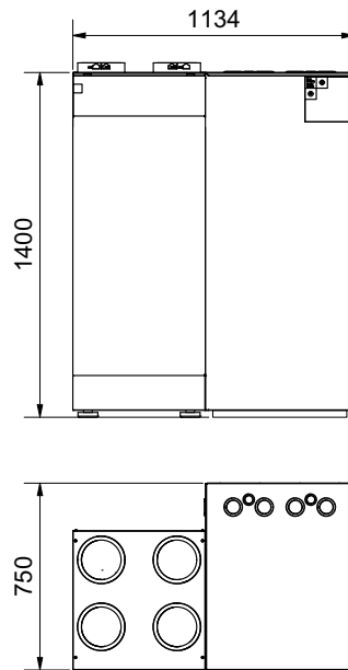
Abb. 6.8:Aufstellbeispiel: System M Comfort
