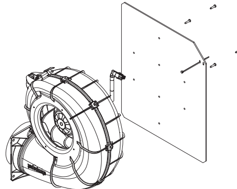
Abb. 11.3: Lüfter rechts
