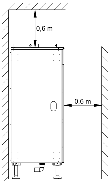
Abb. 6.1: Aufstellung vertikal
