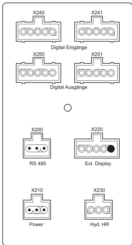
Abb. 6.16: Rückseitige Geräteanschlussplatte
