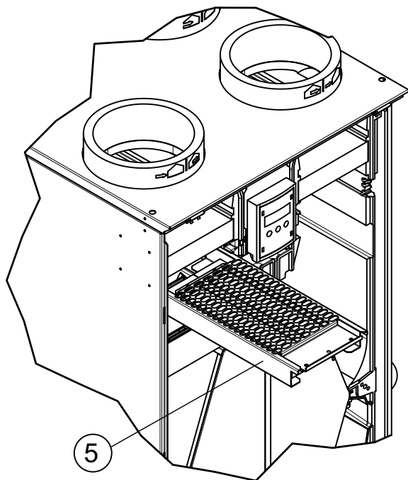
Abb. 5.1: Lüftungsgerät-Ausschnitt mit Vorheizregister
