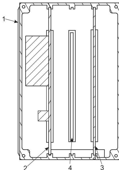
Abb. 6.17: Elektronikbox
