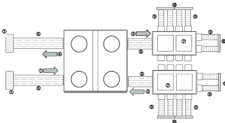
Abb. 6.15: Luftkanalsystem (schematisch, dargestellt für „rechtes Gerät/Zuluft-Anschluss rechts“)
