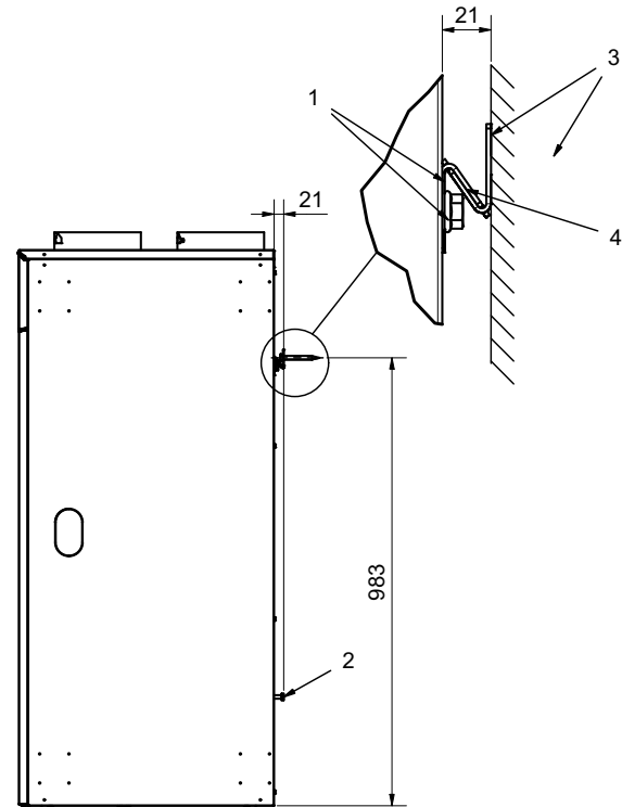
Abb. 6.12:Montage Wandaufhängung
