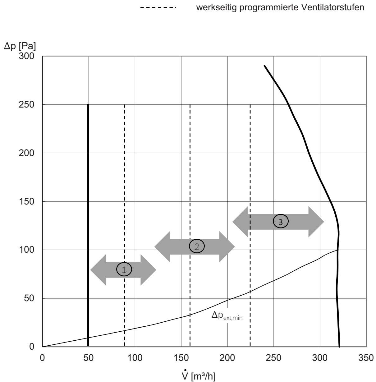
Abb. 15.1: Kennlinie M Flex Air
