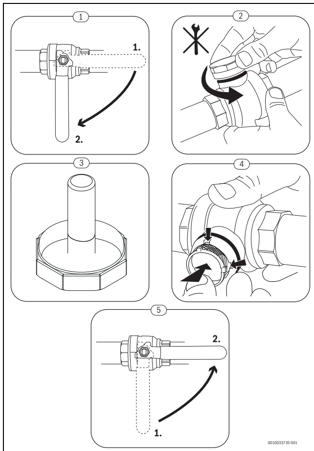
Bild 14 Siebreinigung
