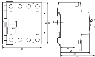
Maßzeichnung Gruppenansicht
