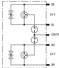
Prinzipschaltbild DPI CD EXI+D 2X24 M
