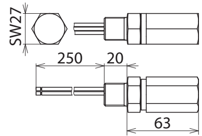
Maßbild DPI CD EXI+D 2X24 M
