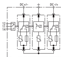
Principalschaltbild DG M YPV SCI 150 FM
