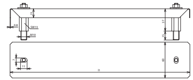
Maßbild AD PAS 10AP V2A
