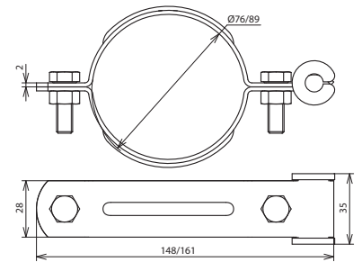
Maßbild LH KD 8.10 D89 STTZN
