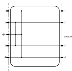
Prinzipialschaltbild BXT M4 E
