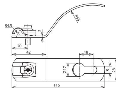
Maßbild DLH DQ 6.10 WPRO5 STTZN
