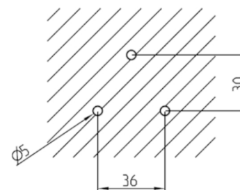
Bohrbild
