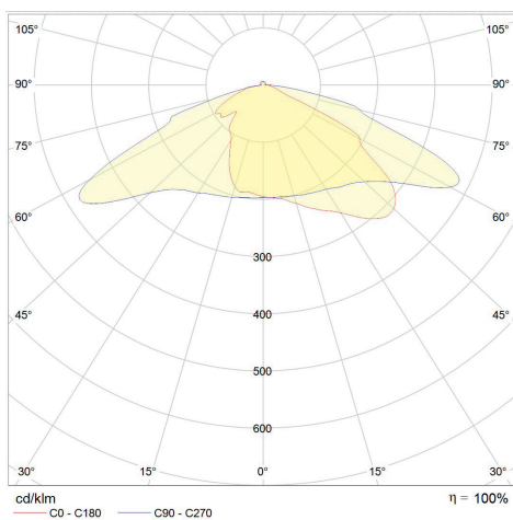
Polardiagramm 150 x 65
