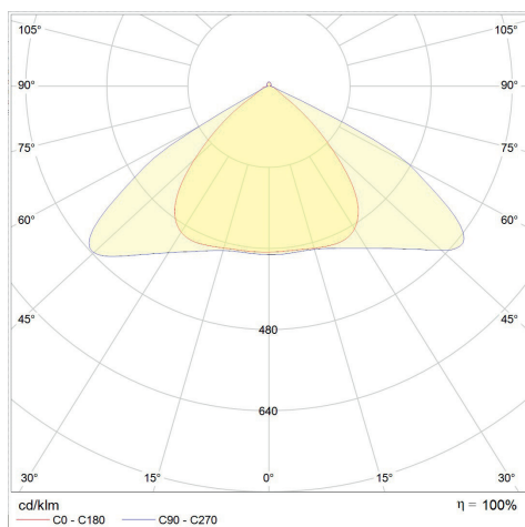
Polardiagramm 120 x 90
