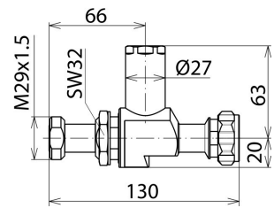
Maßbilder DGA L4 7 16 MFA
