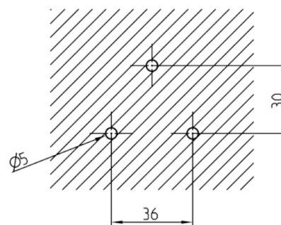
Bohrbild
