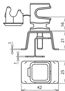
Maßbild LH ZS 8 H16 KB4.16 GR V2A
