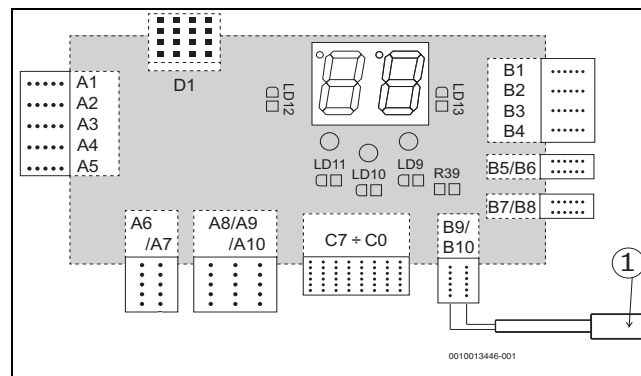
Фиг. 6 Свързване на датчика към клеми B9/B10
