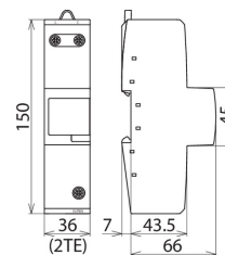
Maßbild DBM 1 440
