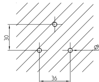
Bohrbild
