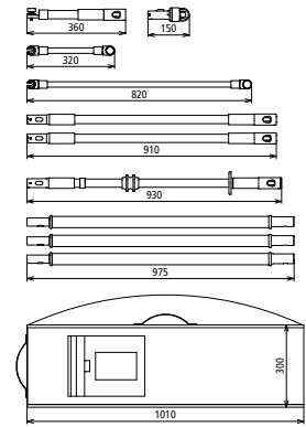
Maßbild ASSN 36 STK ZK
