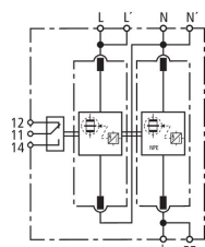
Prinzip Schaltbild DV M TT 2P 255 FM
