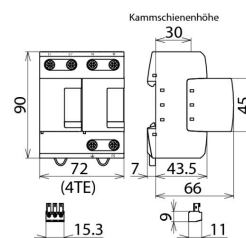
Maßbild DV M TT 2P 255 FM
