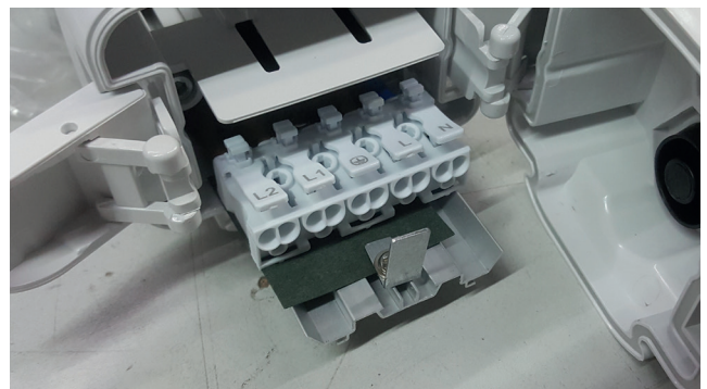
Abb. 5: Lösen der Endkappe, Anschlussraum
