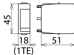
Maßbild DG MOD PV 500
