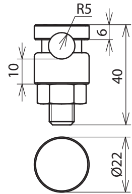
Maßbild KSV 6.10 V4A
