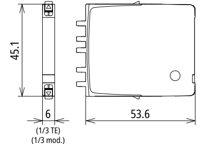
Maßbild BCO MOD ML2 MVG 230
