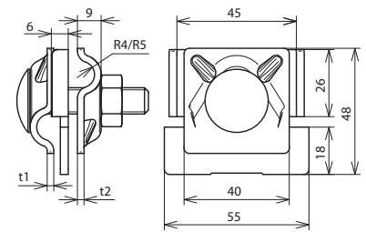
Maßbild
