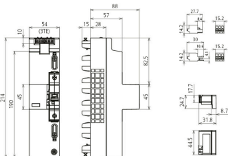
Maßbild DSH ZP 2 LSG A TT 255
