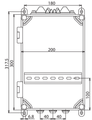
Maßbild IGA 10 V2 IP54
