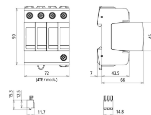
Maßbild DG MD H TT 275 FM
