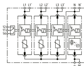
Prinzipialschaltbild DG MD H TT 275 FM
