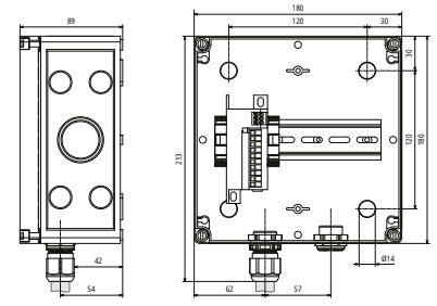
Maßbild DCU EMOB 2 25
