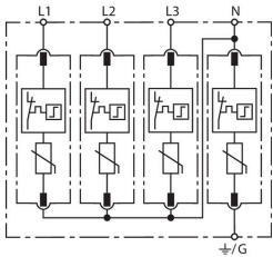
Prinzipialschaltbild DG MU 3PY 208 4W+G
