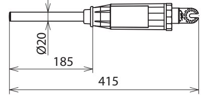
Maßbild PHE3 PK6 20 L SB ZK
