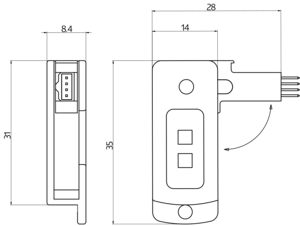
Bemaßung 92684
