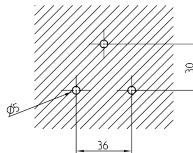
Bohrbild
