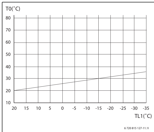
Bild 3 Fußbodenheizung
