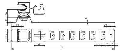
Maßbild DLH US 8 H36 L475 GR V2A
